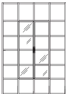
WVS 22 – Kollektion 12, Seite 10 Breite: 155 cm – Höhe: 220 cm – Tiefe: 33 cm
