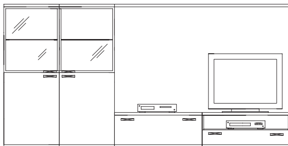
WVS 13 – Kollektion 12, Seite 6 Breite: 333 cm – Höhe: 154 cm – Tiefe: 42 cm / 50 cm
