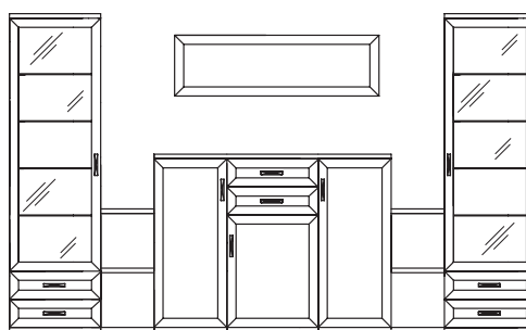
WVS 33 Breite: 346 cm – Höhe: 209,5 cm – Tiefe: 42 cm
